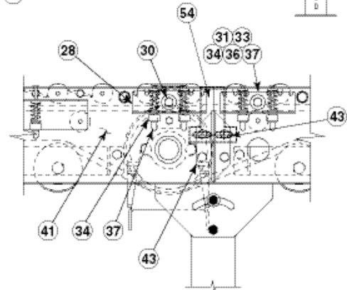
VIEW "A-A" (VISTA "A-A")
